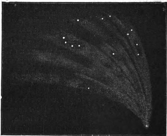
Fig. 38. Comète de 1769.
