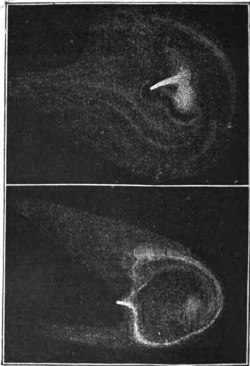
Fig. 41. Comète de 1862. Aspect de la tête.
