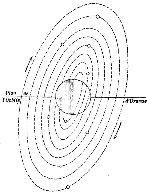
Fig. 35. Uranus.
