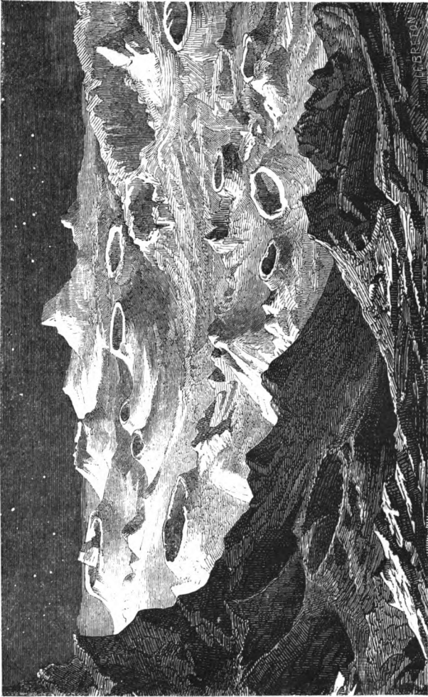
Fig. 47. Paysage lunaire.
