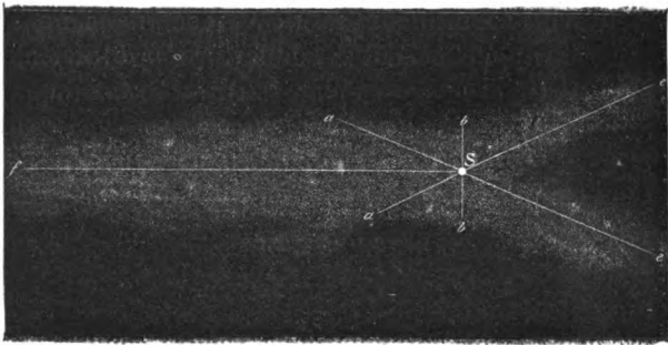
Fig. 13. La Voie lactée.
