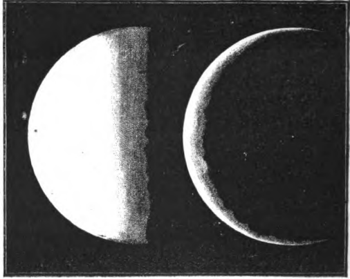
Fig. 30. Échancrures du croissant de Vénus.
