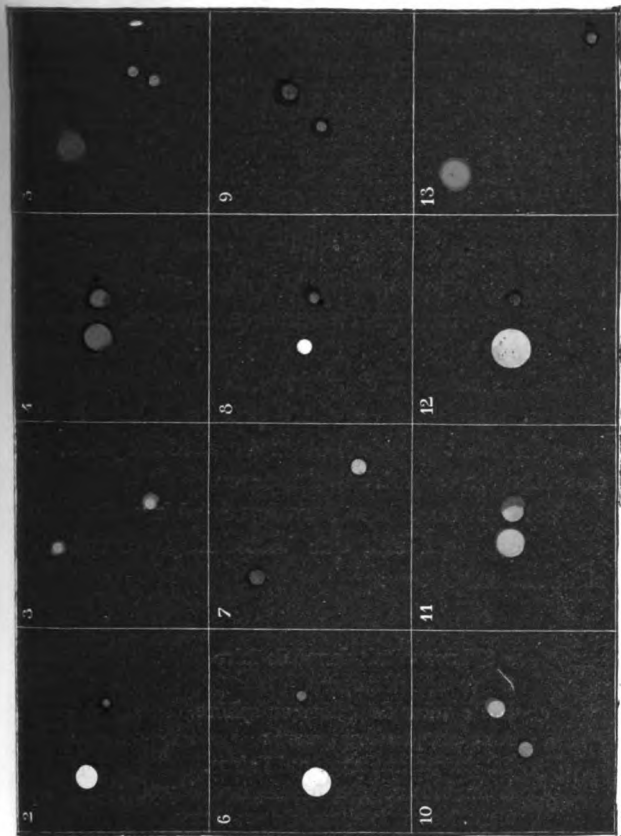
Fig. 24. Etoiles multiples colorées.
