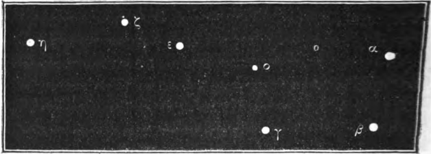
Fig. 14. Constellation de la Grande Ourse.
