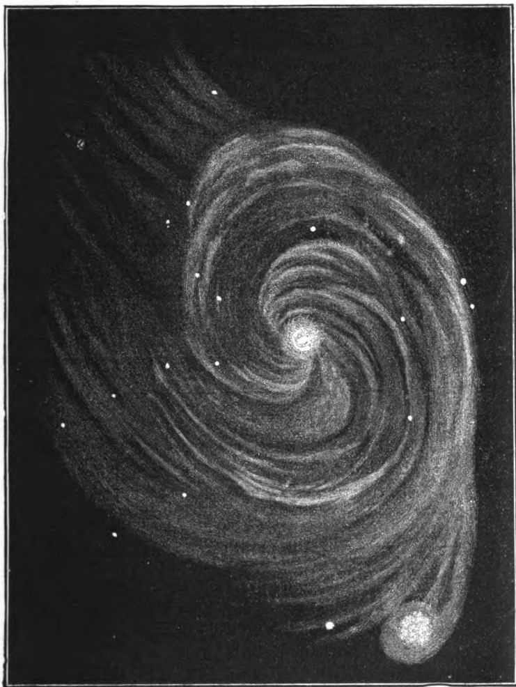
Fig. 11. Nébuleuse des Chiens de chasse.
