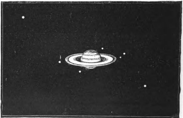
Fig. 33. Saturne et ses satellites.
