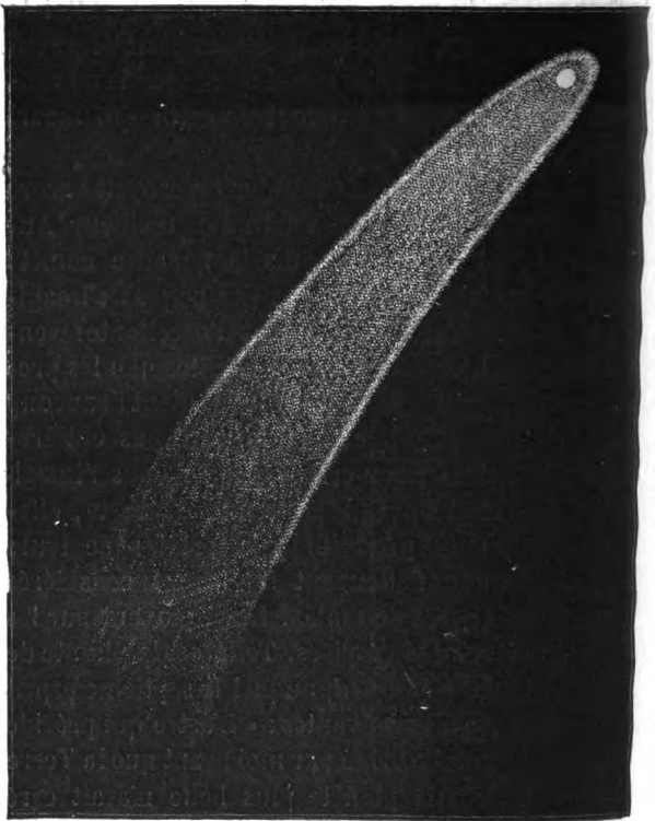
Fig. 39. Comète de 1811.
