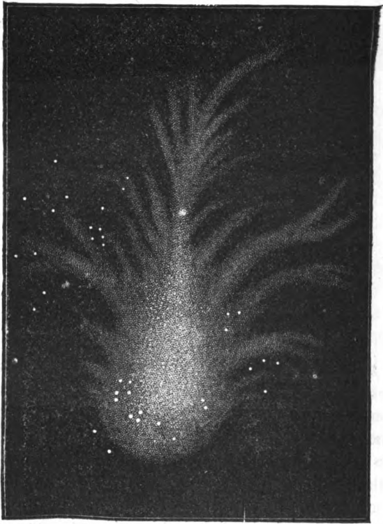
Fig. 7. Nébuleuse du Taureau.
