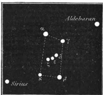
Fig. 20. Orion, Aldébaran, Sirius.
