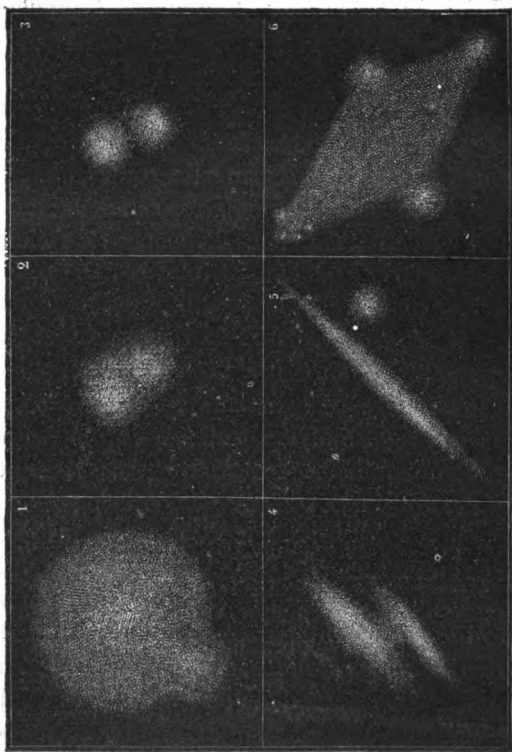
Fig. 10. Nébuleuses doubles et multiples.
