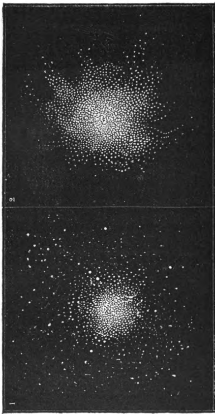
Fig. 4. Amas stellaire.
