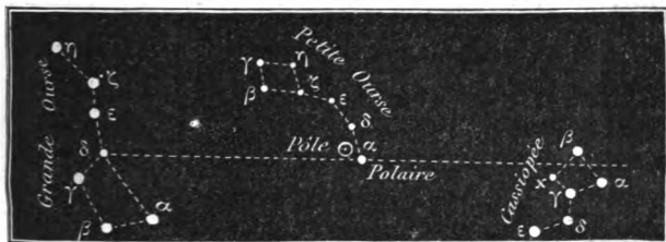
Fig. 15. Grande Ourse, Petite Ourse, Étoile polaire.
