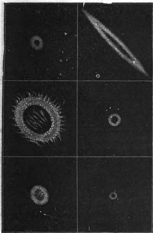
Fig. 5. Nébuleuses annulaires.
