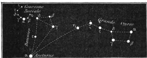
Fig. 18. Couronne boréale, le Bouvier, Arcturus.
