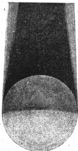
Fig. 1. La nuit et le jour.
