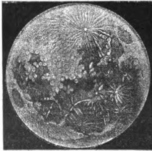
Eig. 48. Aspect de la pleine lune.
