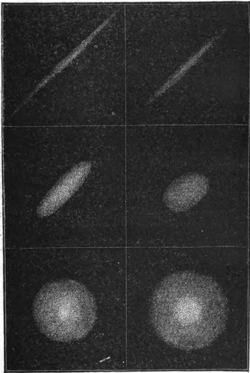
Fig. 3. Nébuleuses globulaires.
