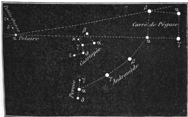
Fig. 16. Cassiopée, Andromède, Pégase.
