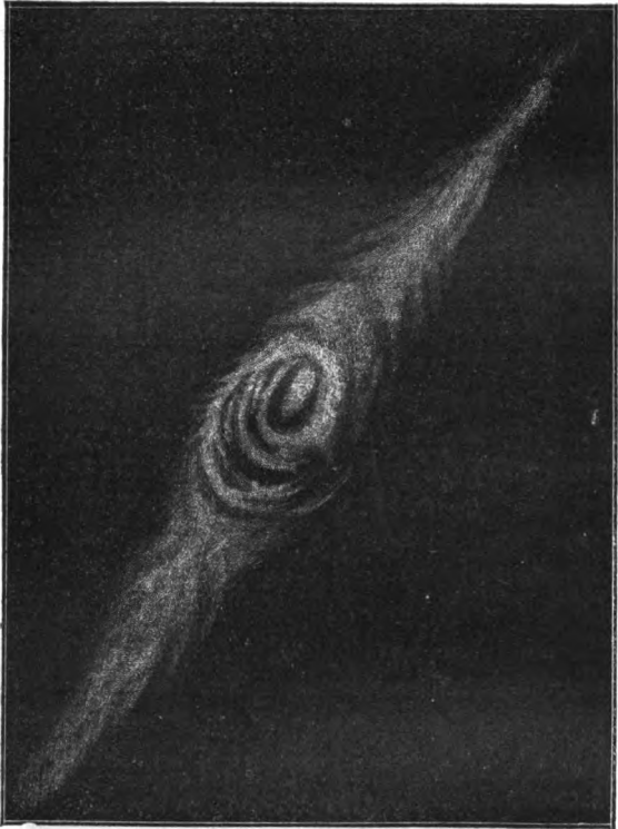
Fig. 6. Nébuleuse du Lion.
